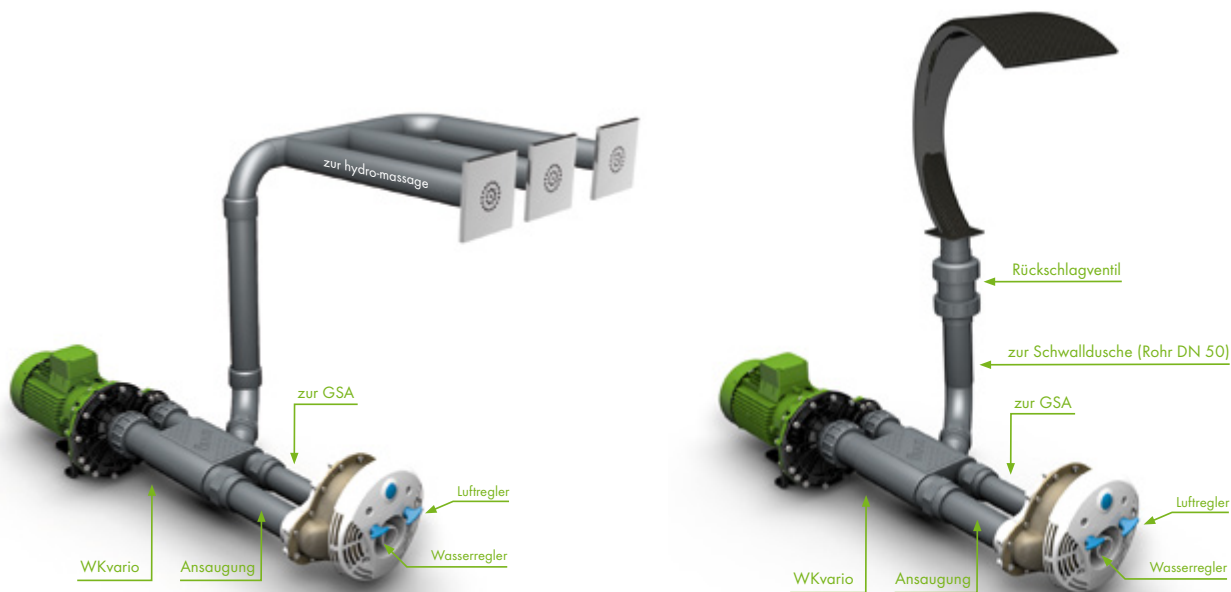
Unverbindliche Systemillustration / Illustration du système, à titre informatif / Suggested installation
