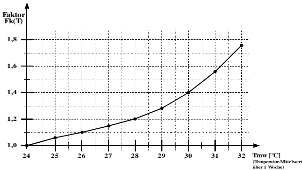
Abbildung 1 Faktor F_k(T)
